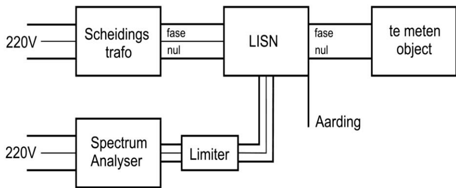
Meten voedingslijnen via LISN 150kHz - 30MHz
